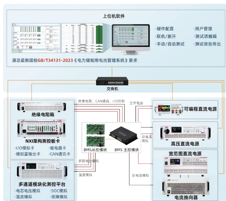
▲ NES6100 系统架构
