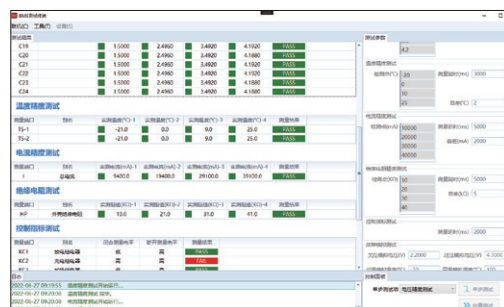
▲ 电流、温度、绝缘电阻测试
