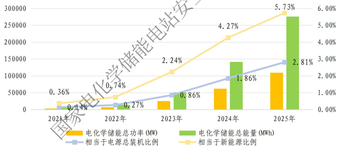
图 1-1 “十四五”时期电化学储能发展情况
