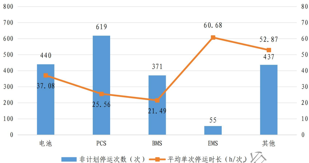
图 4-2 2025 年电化学储能非计划停运情况
