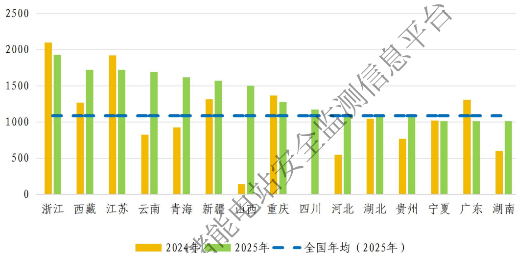
图 2-6 典型区域电化学储能年均利用小时数
