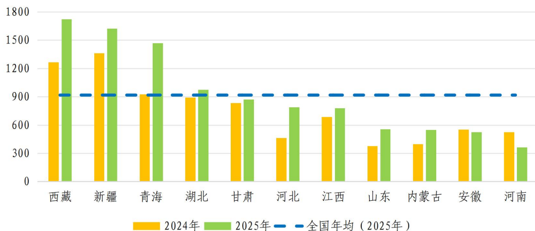
图 2-7 典型区域新能源配储年均利用小时数
