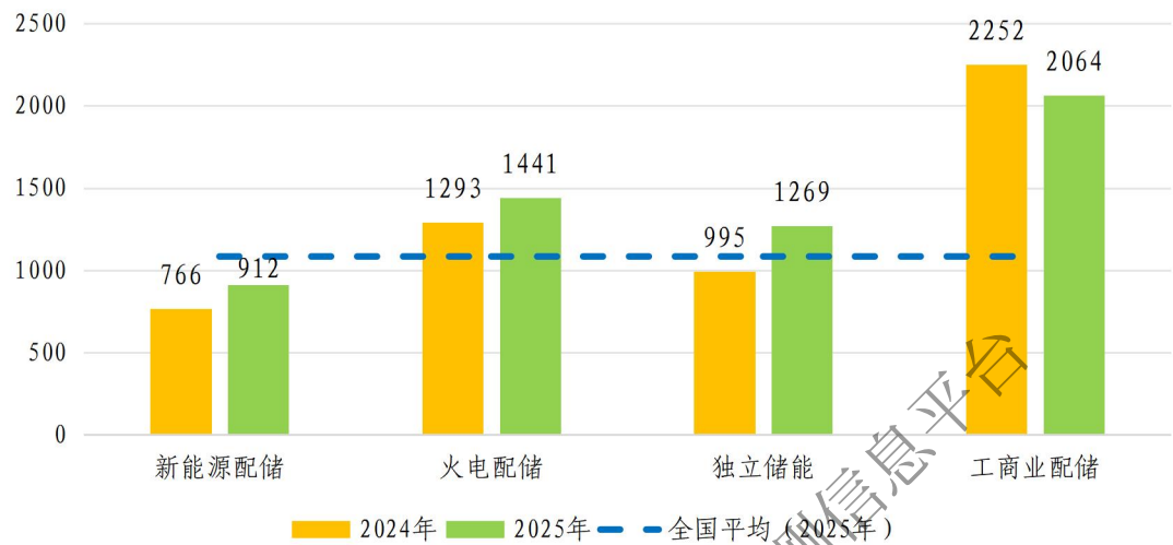
图 2-1 典型应用场景下电化学储能年均利用小时数
