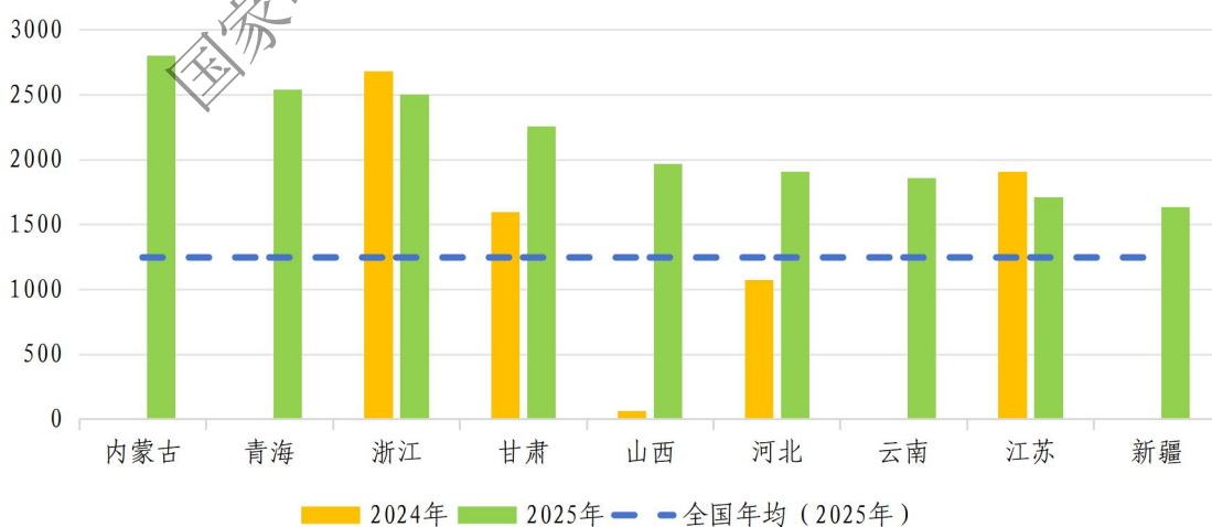
图 2-8 典型区域独立储能年均利用小时数
