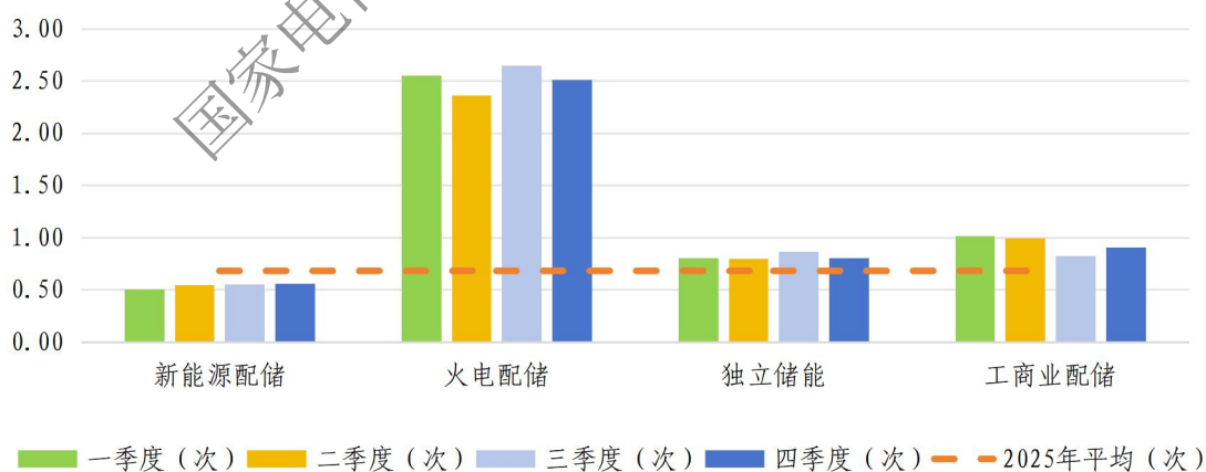
图 2-5 典型应用场景下电化学储能各季度日均等效充放电次数
