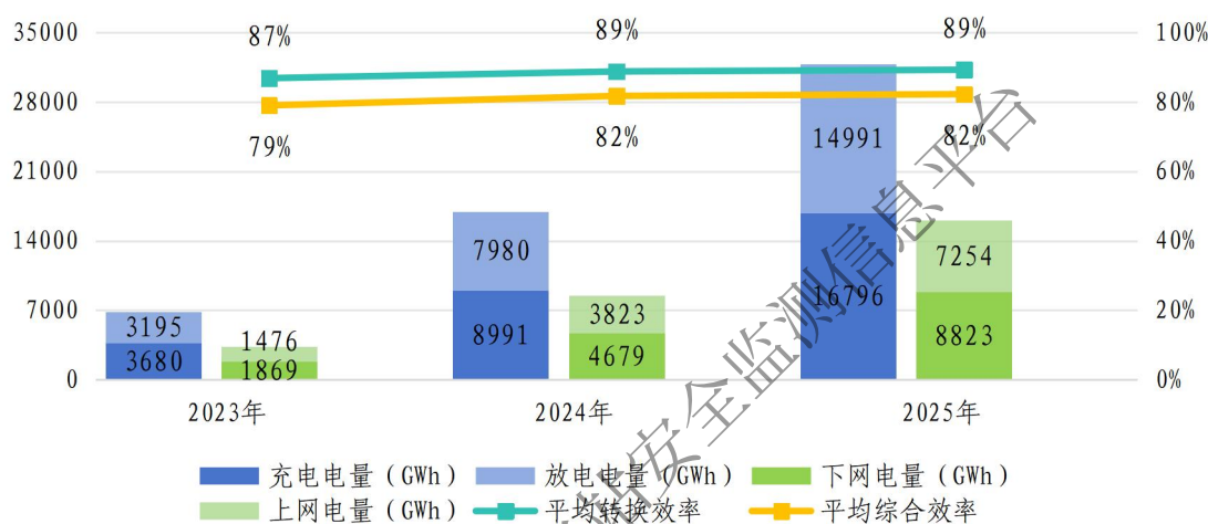
图 3-1 近 3 年电化学储能能效情况
