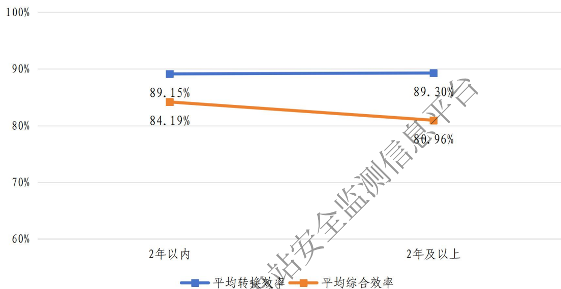
图 3-2 2025 年各投运年限下电化学储能电站能效情况
