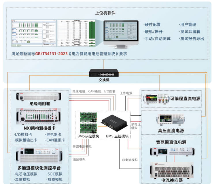
▲ NES6100 系统架构
