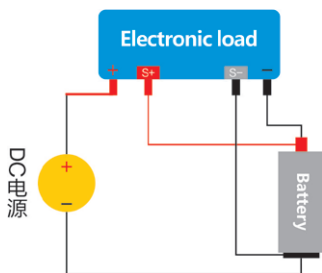
▲ 充电接线图
